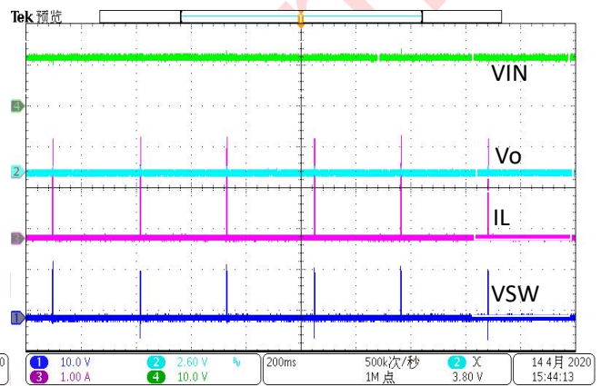
12V 短路保护状态波形图
