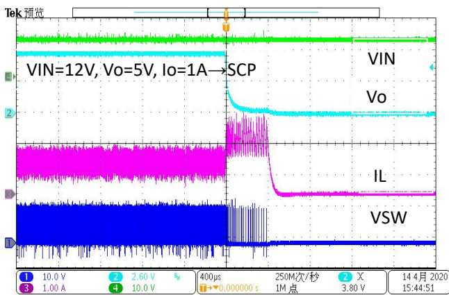
12V 稳态→短路波形图
